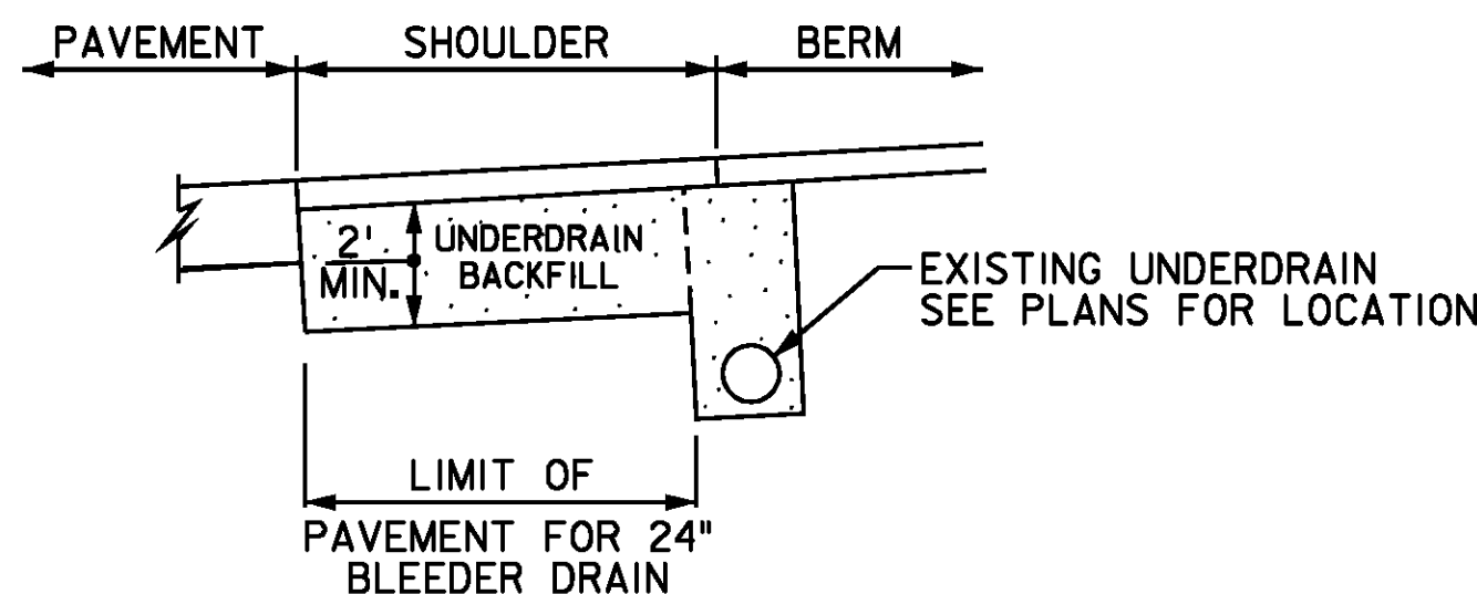
SECTION D-D
